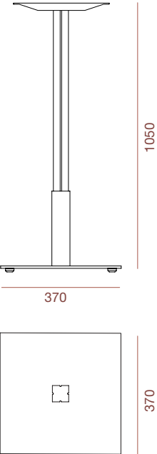
BAR TABLE BASE
