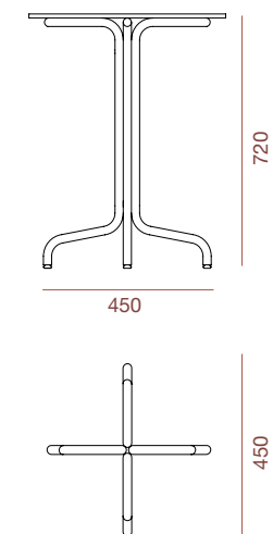
T-4 TABLE BASE
