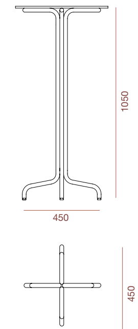
T-4 BAR TABLE BASE
